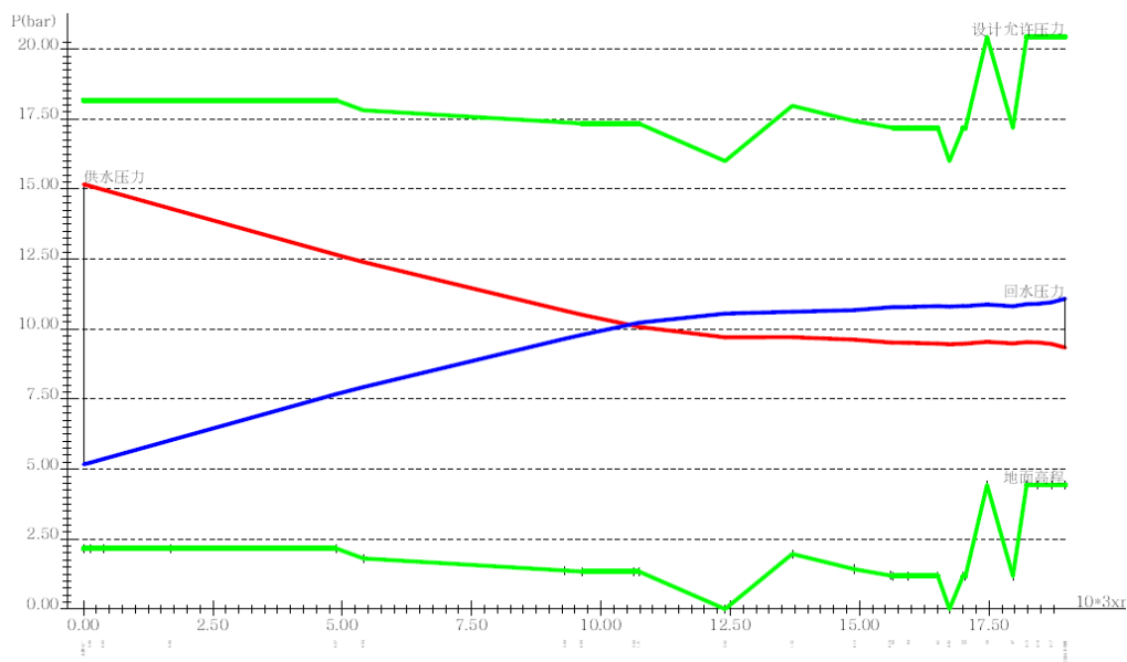
满负荷时水压图
