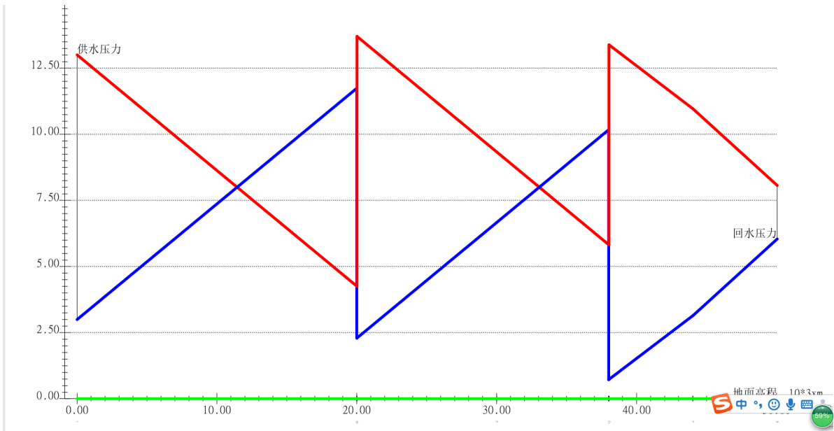
水压图
